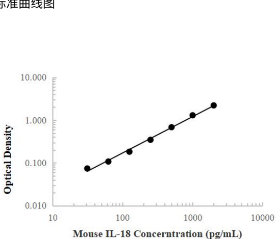
标准曲线图
